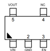
SOT-23-5
