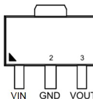
SOT-89-3
