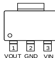
SOT-89-3 ( L-Type )
